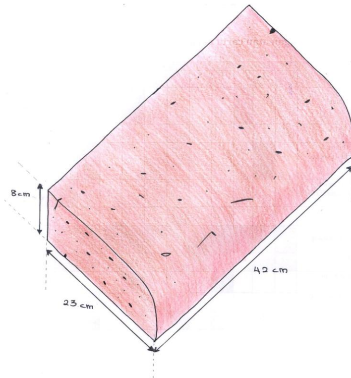
Rajah 3. Lakaran bata separa melengkung.
