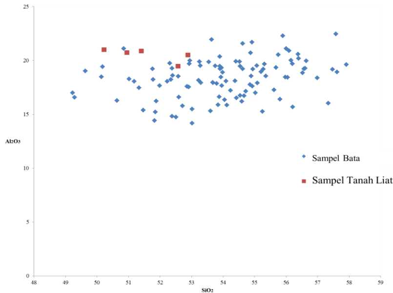
Rajah 4. Kandungan peratusan berat kering SiO 2 dan Al 2 O 3 dalam sampel bata dan lempung di sekitar kawasan percandian.
